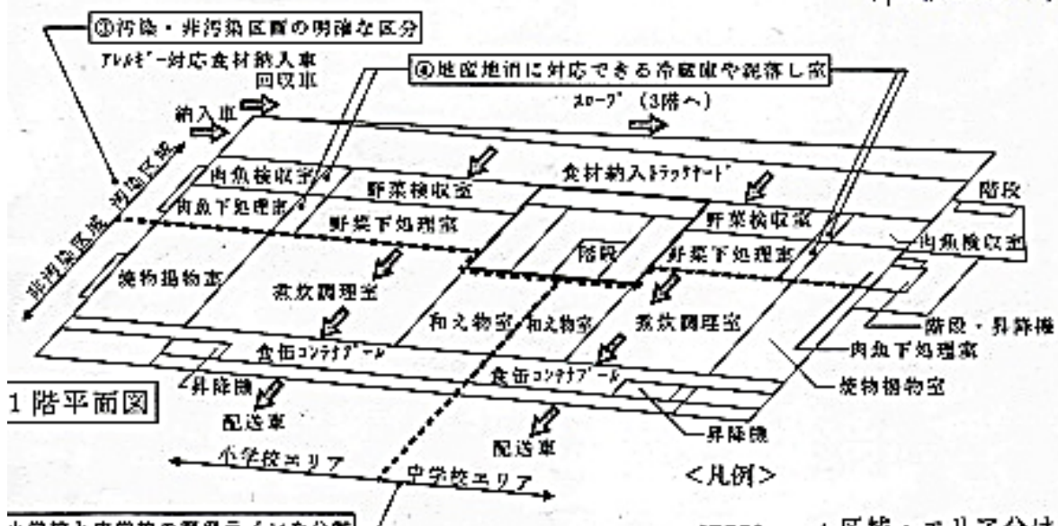
平面図 1 : 600
